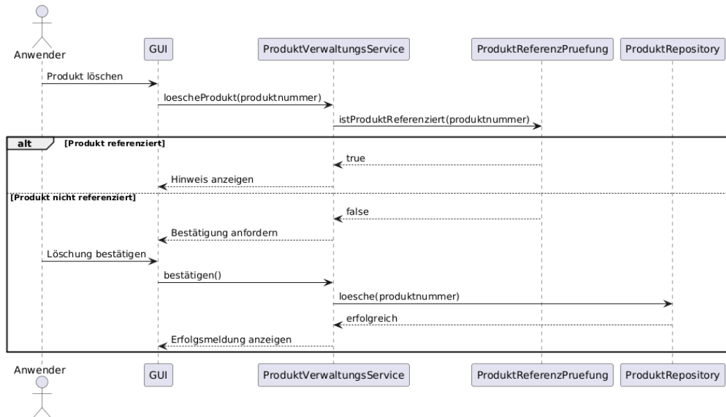
Abbildung 2: UML-Sequenzdiagramm „Produkt löschen mit Löschsperre“ (Gruppe B)
