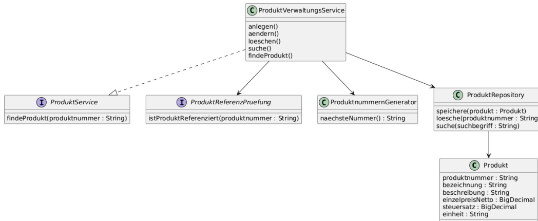
Abbildung 1: UML-Klassendiagramm Produktverwaltung (Gruppe B)
