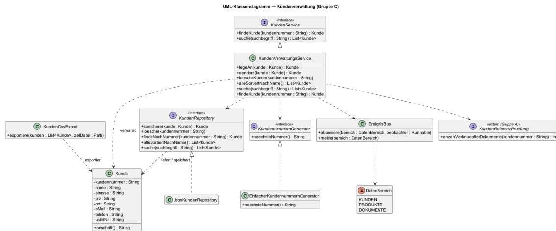
Abbildung 1: UML-Klassendiagramm Kundenverwaltung
