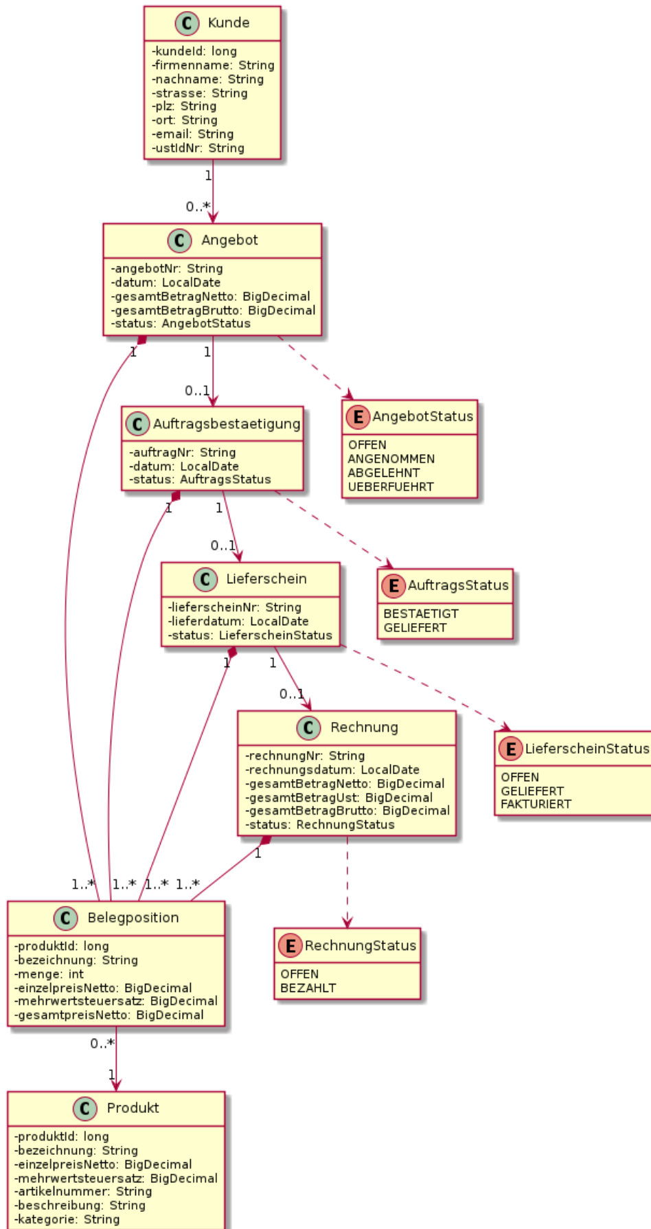
Abbildung 3: UML-Klassendiagramm der Datenobjekte mit Java-Typen und Multiplizitäten.
