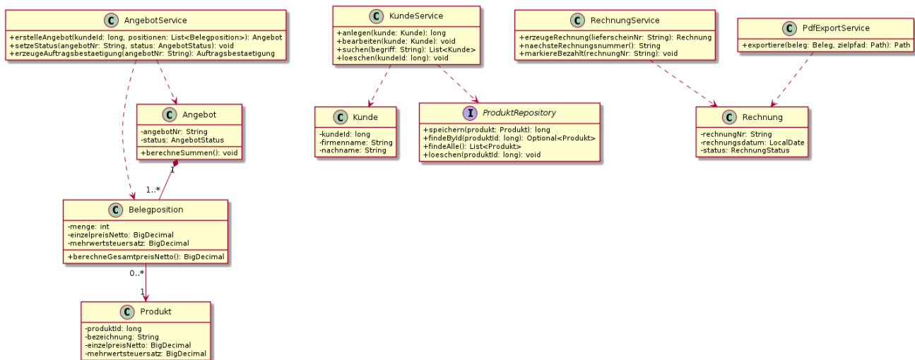
Abbildung 4: Abbildung 5: Detailliertes UML-Klassendiagramm der Kernklassen mit Methodensignaturen.
